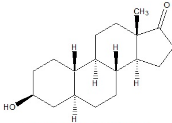
5alpha-Estran-3beta-ol-17-one
