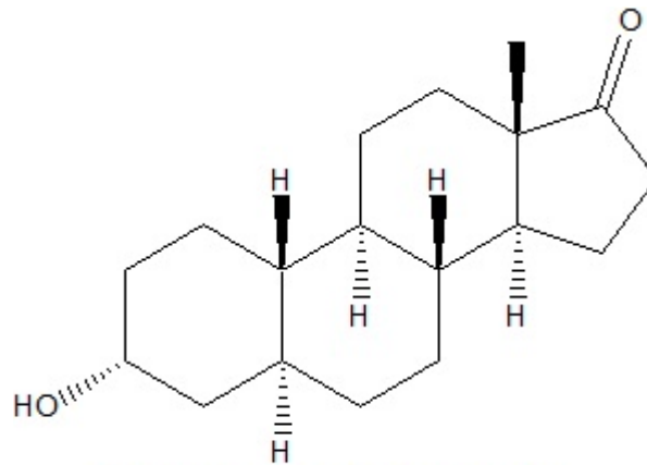
5alpha-Estran-3alpha-ol-17-one
